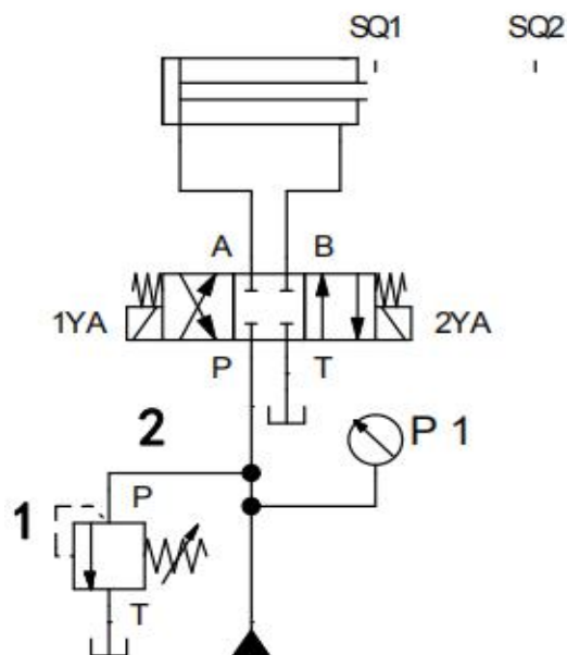
图 J1-3 自动连续换向回路的液压回路
