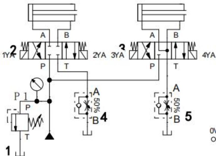
图 J1-9 回油路采用调速阀控制双缸同步回路的液压回路
