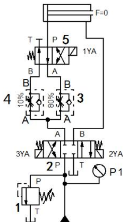
图 J1-6 并联调速回路调速阀的液压回路
