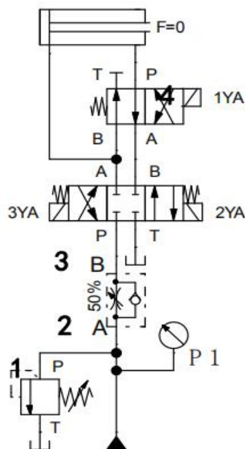
图 J1-4 差动连接工作进给快速回路的液压回路
