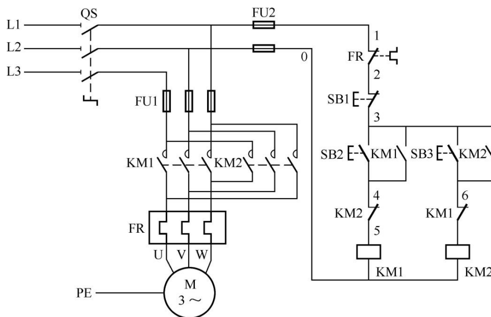
图 K1-4 继电器控制系统的原理图与制作参考图
