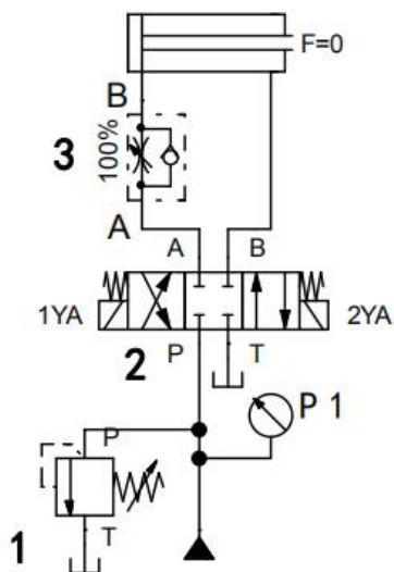
图 J1-1 进油路节流调速回路的液压回路
