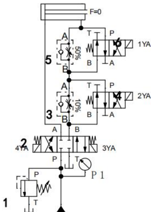
图 J1-10 调速阀串联多级调速回路的液压回路
