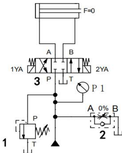
图 J1-2 节流阀旁路节流调速回路的液压回路
