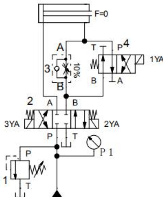
图 J1-5 调速阀短接调速回路的液压回路
