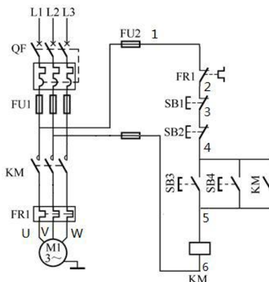
图 K1-2 系统的原理图与制作参考图
