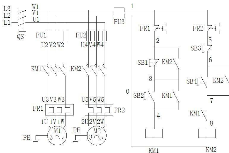
图 K1-8 继电器控制系统的原理图与制作参考
