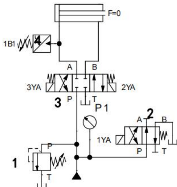
图 J1-8 压力继电器控制液压缸动作及卸荷回路的液压回路
