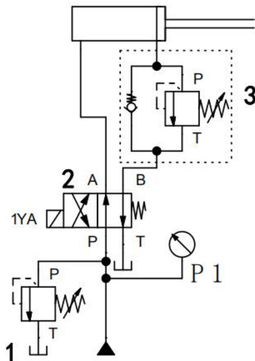
图 J1-7 采用单向顺序阀控制液压缸的平衡回路
